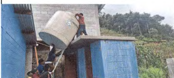
Foto 10: Colocación de depósito de agua en el lugar correspondiente.
